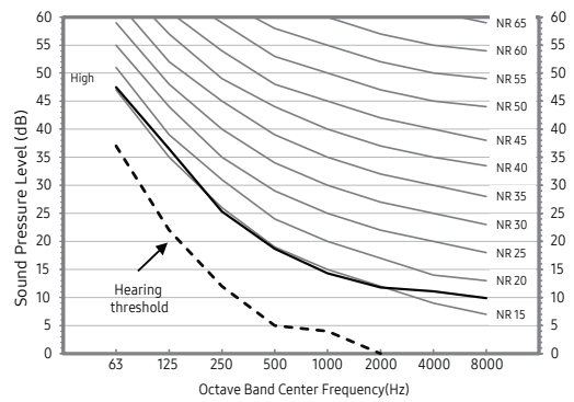
2) AE260RNWSEG/EU + AE060RXEDEG/EU
